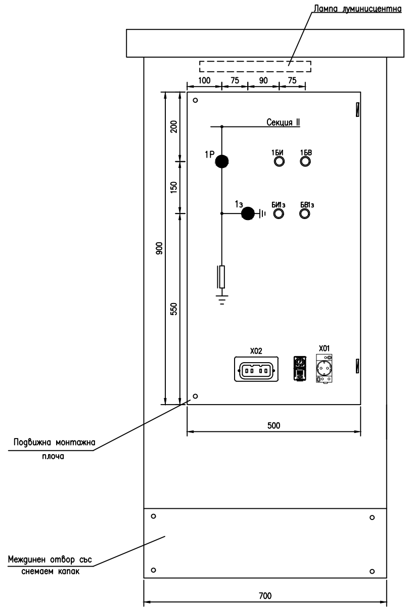
Поглед при отворена външна врата Разположение на апаратурата
