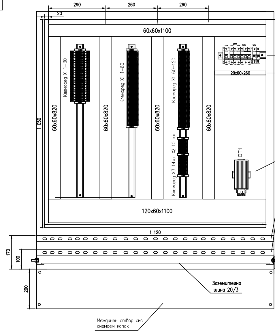
Поглед при отворена външна врата Неподвижна монтажна плоча
