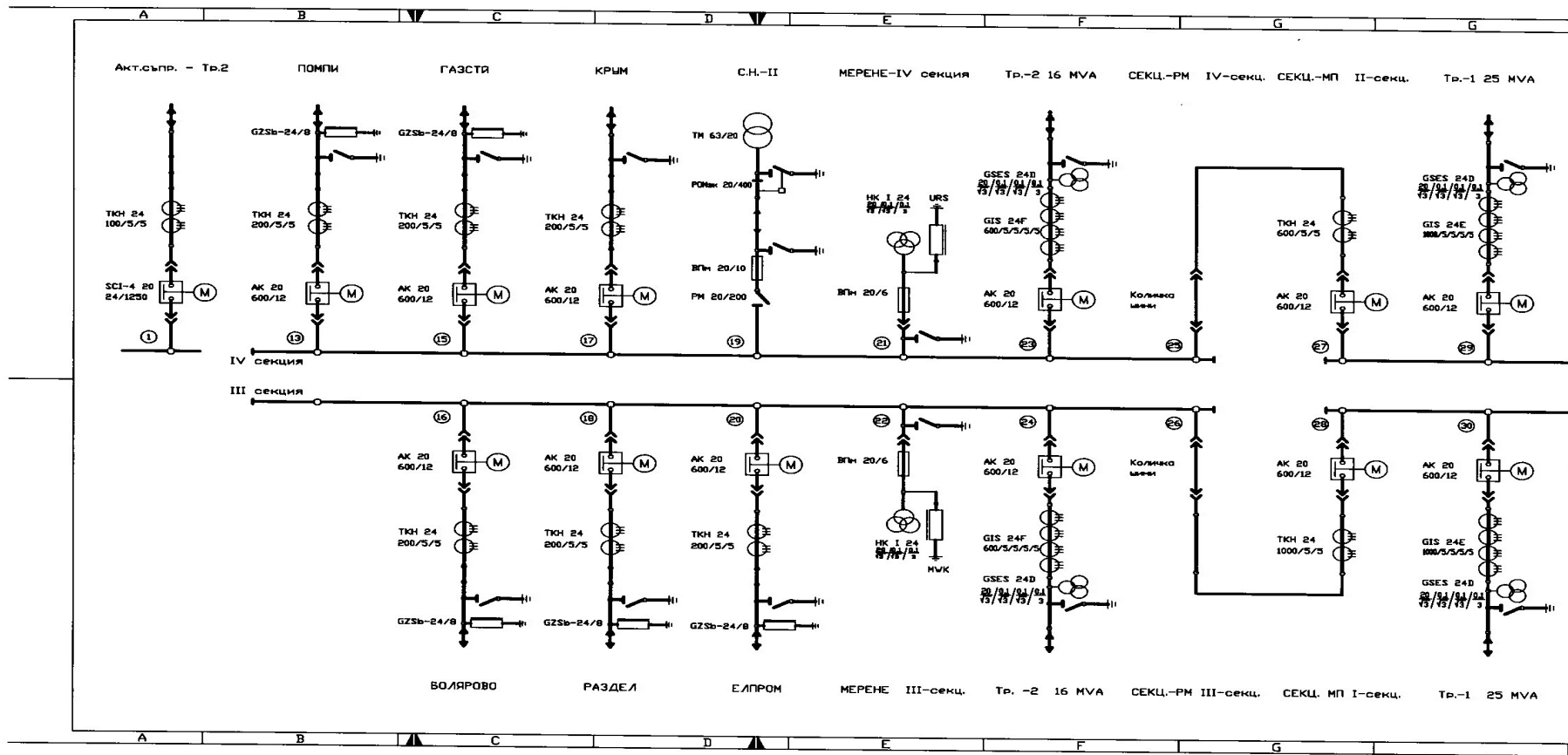
фиг. 1.2. Еднолинейна схема на п/ст „Елхово“, III и IV секция
